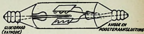
DE OUDSTE TRIODE DOOR PHILIPS IN DE HANDEL GEBRACHT
