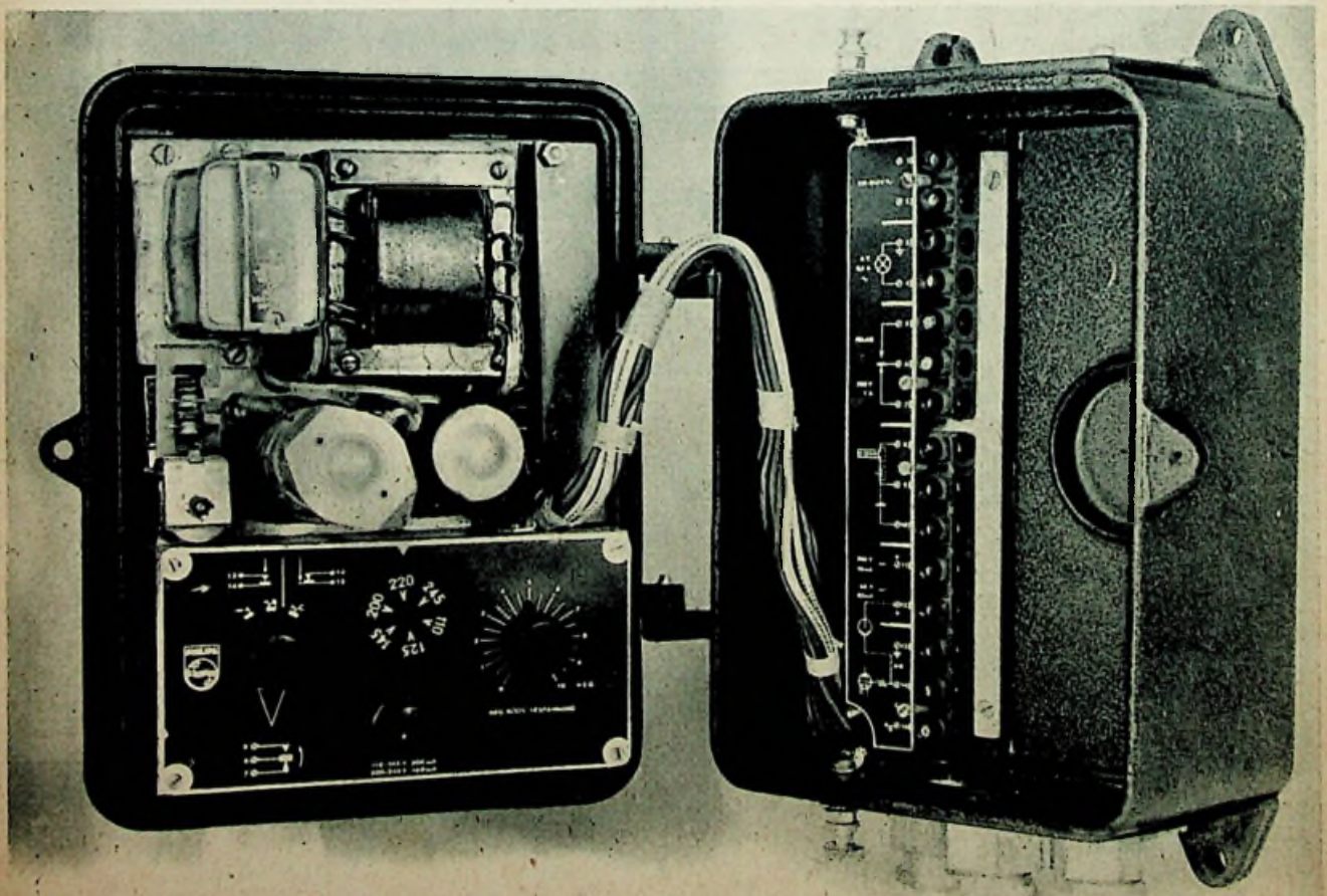
Relaisbuischakelapparaat
