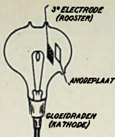
DE TRIODE IN EEN VAN ZIJN OUDSTE VORMEN
